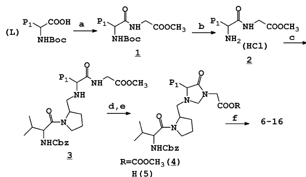
Scheme 1. (a) IBCF/NMM then Gly-OCH 3 (HCl); (b) HCl/dioxane; (c) Cbz-L-Val-L-prolinal/NaBH (OAc) 3 ; (d) 37% aq HCHO; (e) aq KOH; (f) CDI/THF then RNH 2 .
